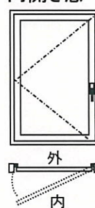
内開き窓
